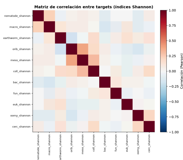
Figura 14: Gráfica de correlación de los índices Shannon.
